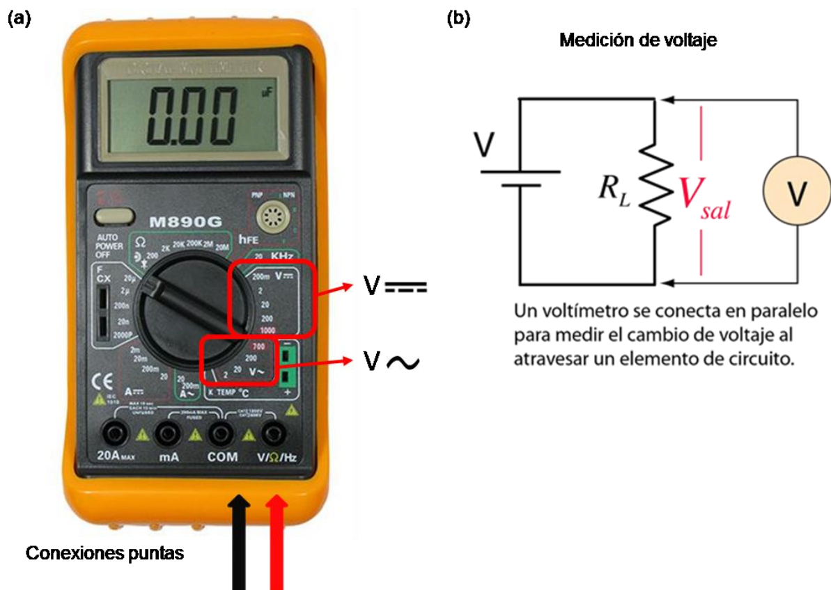
Figura 2: configuración para función de medición de voltaje.
