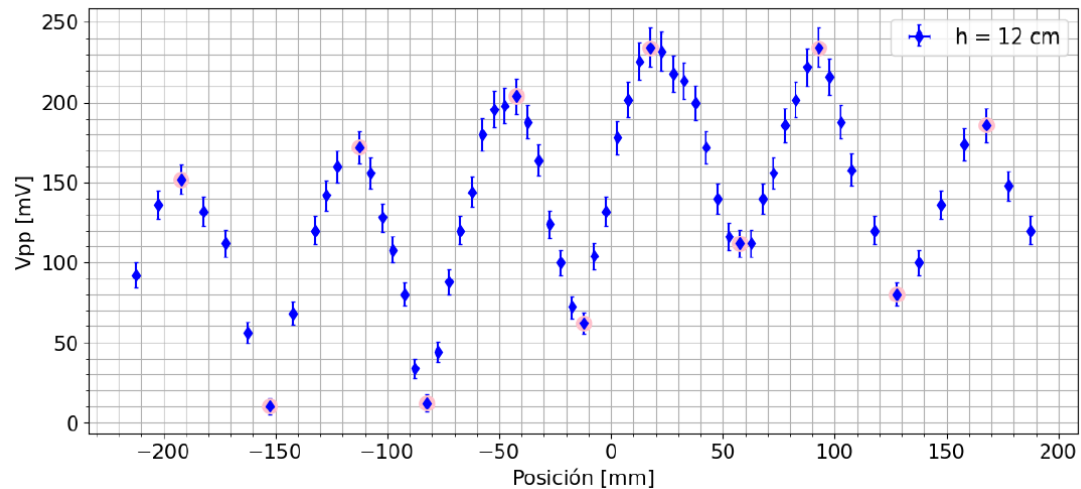
Medición de interferencia medida en el laboratorio ( h = 12 \text{ cm} , f = 39 \text{ kHz} )
